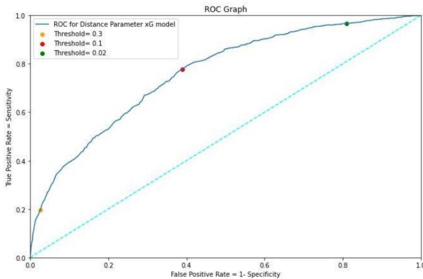
Fig. 21. ROC Graph for Distance Parameter xG Model
