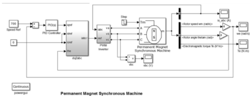
Gambar 8. Simulink MSM [5]
