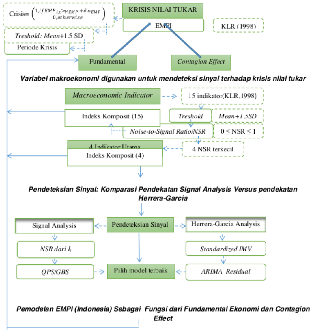
Gambar 4.1: Tahapan Estimasi Model
